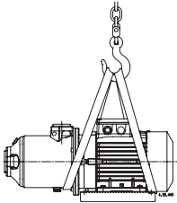
Sollevario pompa Raising the pump Anhebung Pumpe Suolèvement de la pompe Elevación de la bomba 吊起水泵
