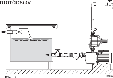
Fig. 1 Funzionamento sotto battente Positive suction head operation Zulaufbetrieb Fonctionnement en charge Funcionamiento bajo carga 正吸水水头的操作
