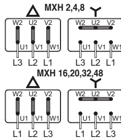
Schema elettrico Electrical diagram Schaltbild Schéma électrique Esquema eléctrico 电气图
